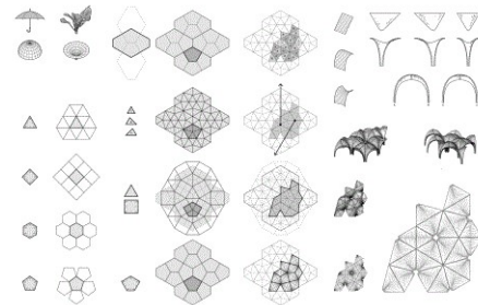
[그림 3-15. 파라메트릭 디자인 사례 43) ]
